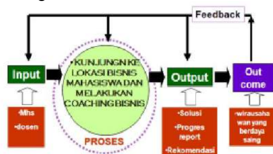
Gambar 6. Konsep Monev
